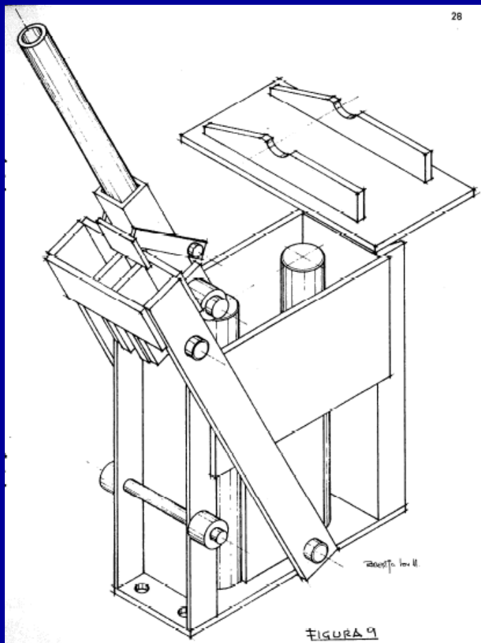
CINVA-RAM
